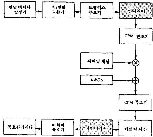
그림 9. 인터리빙 방법을 적용한 트렐리스 부호화된 CPM 변조 시스템
