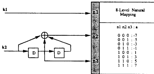
그림 4. r=2/3 인 8레벨 트랜리스 부호화된 CPFSK의 매핑 방법 (K=3, (7, 2)코드)
