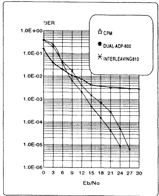
그림 13. 페이딩율 20 Hz에서 이중모드 적응복호와 인터리빙의 성능곡선(메모리 : 800, h = 1/4) Fig. 13. Performance graph of the CPFSK dual mode adaptive decoder (memory : 800, h = 1/4) over the fading channel with the fading rate 20Hz.
