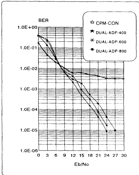
그림 10. 페이딩율 20 Hz에서 CPFSK 이중모드 적응복호의 성능곡선(h=1/4) Fig. 10. Performance graph of the CPFSK (h=1/4) dual mode adaptive decoder over the fading channel with the fading rate 20Hz.
