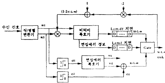
그림 2. (2, 1, m) 부호기를 사용한 적응 복호기 Fig. 2. Adaptive decoder for the (2, 1, m) encoder.
