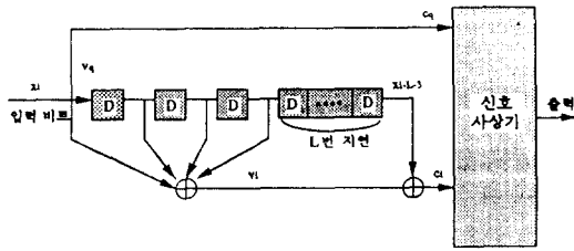
그림 1. (2, 1, m) 이중모드 적응 부호기 Fig. 1. (2, 1, m) Dual mode adaptive encoder.
