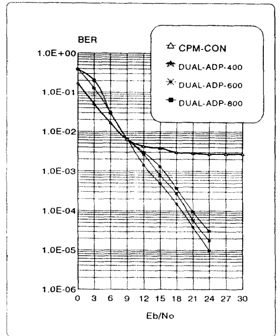
그림 11. 페이딩율 100 Hz에서 CPFSK 이중모드 적응복호의 성능곡선(h=1/4) Fig. 11. Performance graph of the CPFSK (h=1/4) dual mode adaptive decoder over the fading channel with the fading rate 100Hz.
