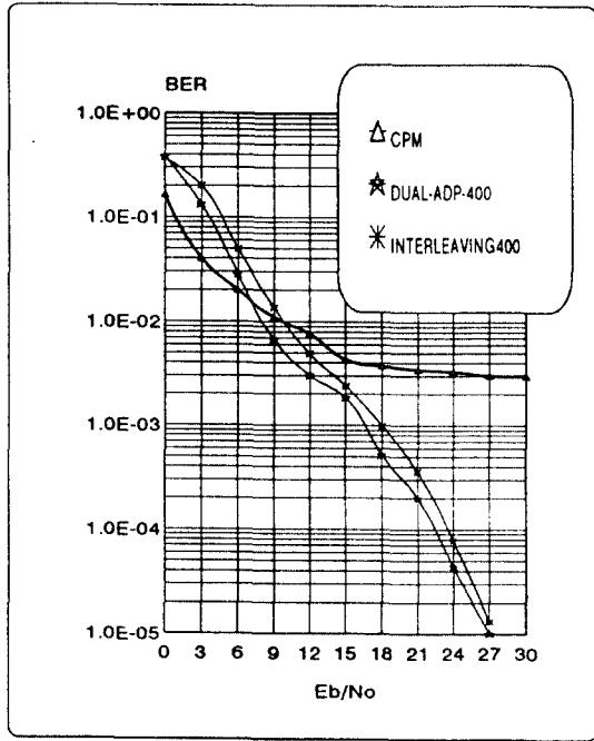
그림 12. 페이딩율 20 Hz에서 이중모드 적응복호와 인터리빙의 성능곡선(메모리 : 400, h = 1/4) Fig. 12. Performance graph of the CPFSK dual mode adaptive decoder (memory : 400, h = 1/4) over the fading channel with the fading rate 20Hz.
