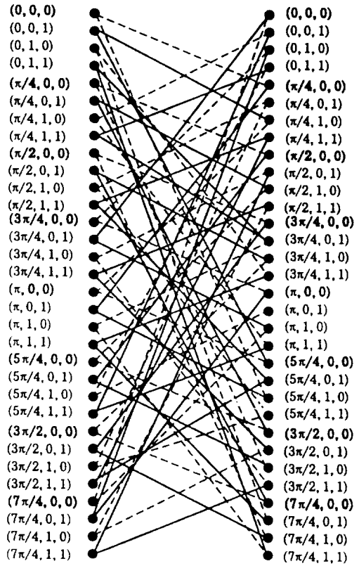
그림 5. 그림 4의 트랜리스 Fig. 5. The trellis structure of Fig. 4.
