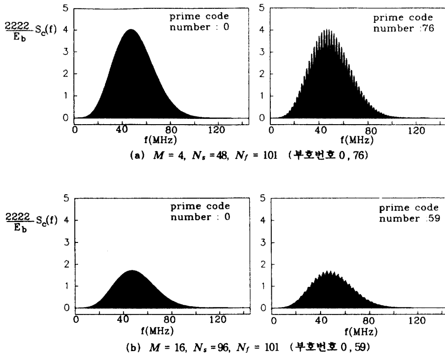
그림 13. 시스템 1의 변조기 출력신호의 연속스펙트럼성분 ( R_b = 10kbps, T_c = 41.254 \mu sec )
