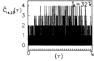
(b) N_f = 41, N_s = 32 인 변형된 소수부호의 상호상관함수(부호번호 14, 23)
