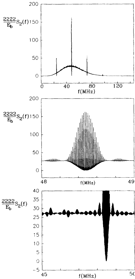
그림 16. 이상 가우시안 무선채널상의 한 지점에 서로다른 부호를 갖는 101명의 동시사용자의 신호들이 같은 전력으로 도달했을 경우 전체 전력스펙트럼 (시스템 2, M=16 , N_f=101 , N_c=96 , R_b=10 kbps, T_c=41.254n sce)
