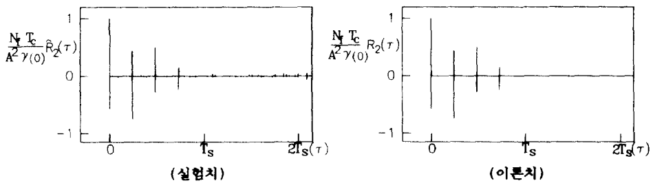
그림 11. 자기상관함수의 이론치와 실험치의 비교(시스템 2) ( M=4, N_s=16, N_f=17 , 부호번호 8)
