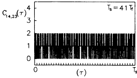
(a) N_f = 41 인 소수부호의 상호상관함수(부호번호 14, 23)
