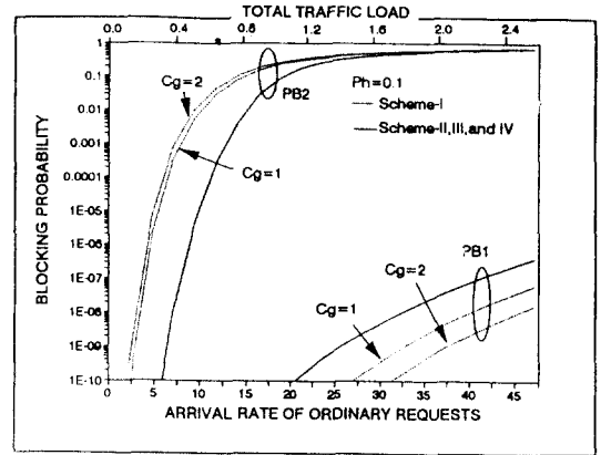
그림 5. Ph = 0.1 일 때 4가지 요청처리방식의 blocking 확률 비교. Fig 5. Comparison of blocking probability of four request handling schemes for Ph = 0.1 .
