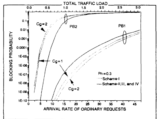
그림 6. Ph = 0.3 일 때 4가지 요청처리방식의 blocking 확률 비교. Fig 6. Comparison of blocking probability of four request handling schemes for Ph = 0.3 .
