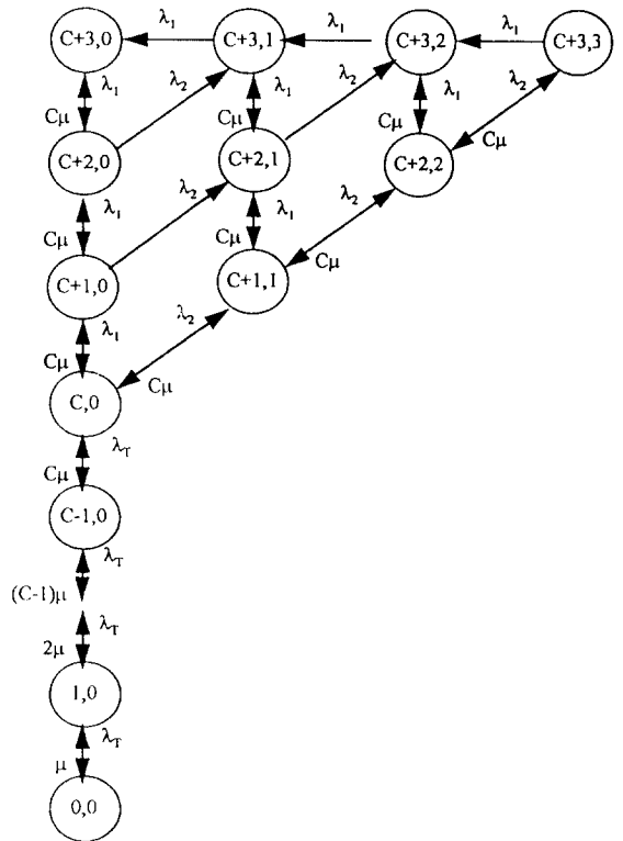
그림 4. 방식II에 의한 상태 천이도( K=C+4 인 경우). Fig 4. State-transition-rate diagram for Scheme-II (for K=C+3 ).
