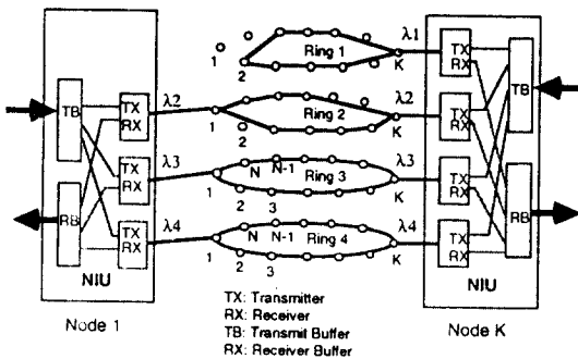
(b) 하이브리드 광섬유 구성의 예 (b) An Example of a Hybrid Channel Configuration.
