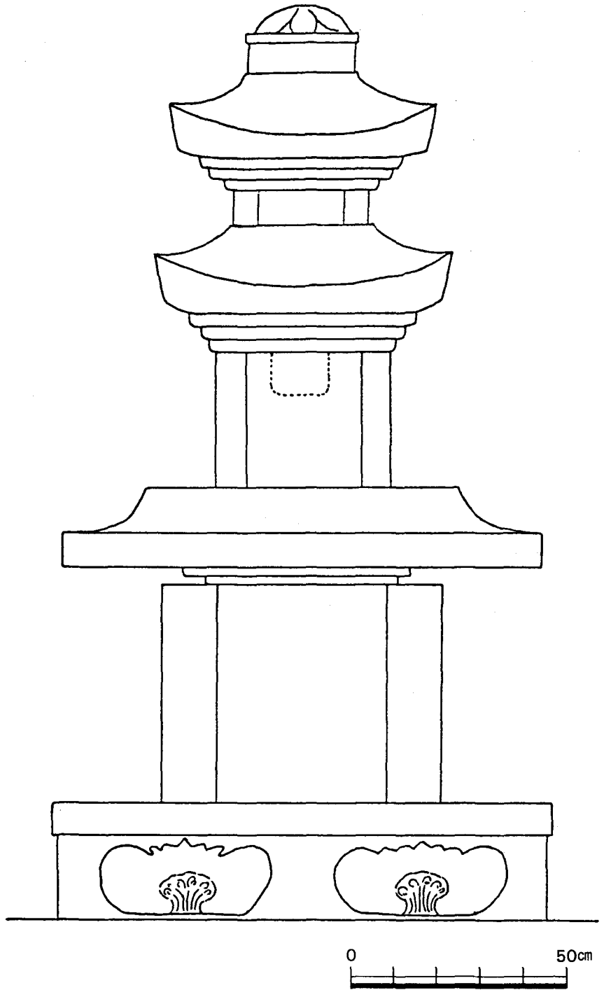
甲屯里 三層石塔 實測圖
