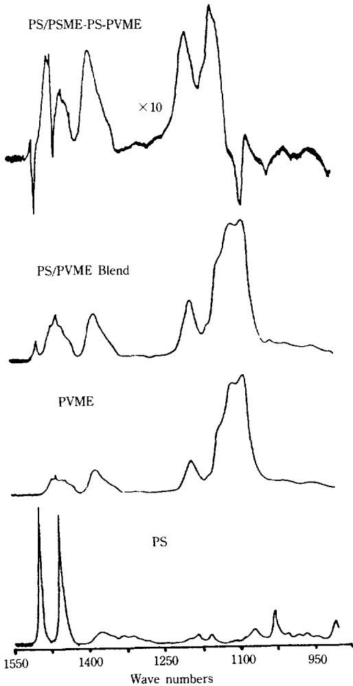
그림 6. PS/PVME : compatible blend ; interaction spectrum.
