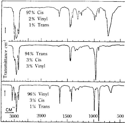
그림 10. Infrared spectra of butadien polymers.
