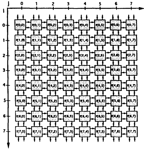
그림 2. (8×8) 2D VR-FCT 구현을 위한 2차원 어레이 및 데이터 매핑. Fig. 2. 2-D array and data mapping for implementing (8×8) 2-D VR-FCT.
