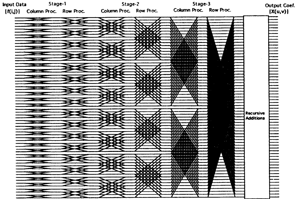
그림 1. (8x8) VR-FCT의 연산흐름도. Fig. 1. The signal flow graph for (8x8) VR-FCT.
