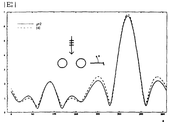
그림 2. 두개의 유전체 실린더에 의한 산란전계 Fig 2. The scattered field pattern from two identical dielectric cylinders
