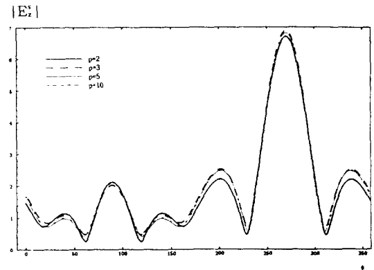
그림 3. 두개의 유전체 실린더에 의한 산란전계( p=2, 3, 5, 10 ) Fig 3. The scattered field pattern from two identical dielectric cylinders( p=2, 3, 5, 10 )
