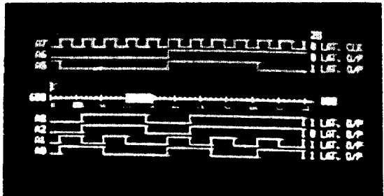
사진 3. ROM을 통과한 후의 데이터 래치 Photo 3. Data latch after the ROM
