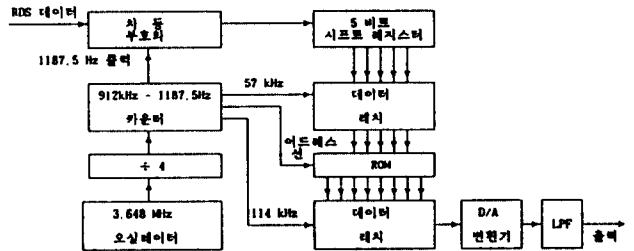
그림 8. 송신단의 하드웨어 장치 Fig. 8. Hardware device for the transmitter
