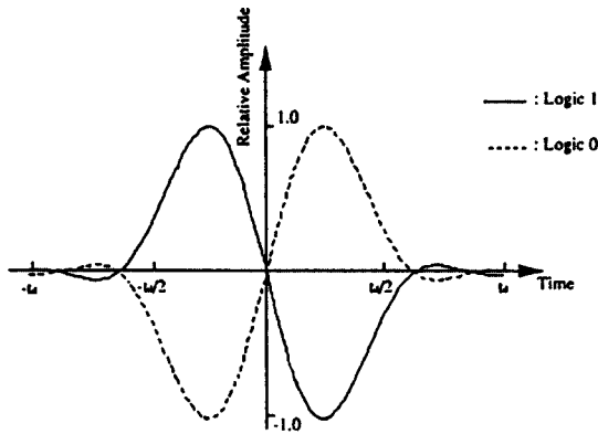
그림 3. biphasе 심볼의 시간 함수 Fig. 3. Time function of biphasе symbol
