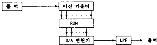
그림 6. 디지털 파형 여파기의 구조 Fig. 6. Configuration of the digital waveform filter
