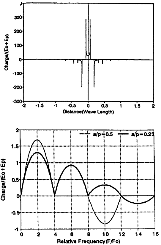
그림 2. 기본 전하분포 함수 Fig 2. Basic Charge Distribution function
