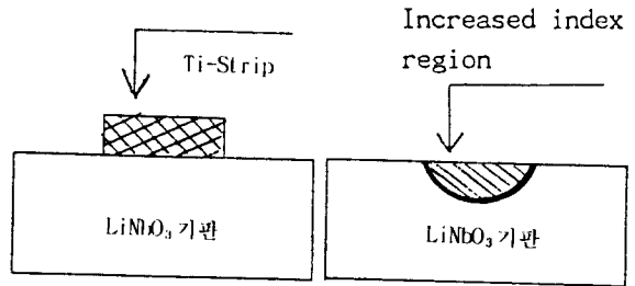
그림 1. Ti 내부 확산 방법 Fig. 1. Titanium-indiffusion method.
