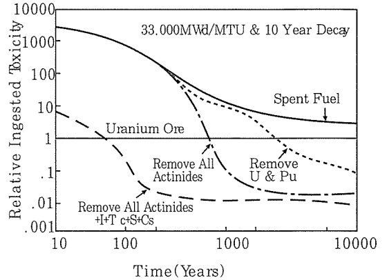
그림 1. 사용후 핵연료와 소멸처리후 방사성폐기물의 시간에 따른 독성비교
