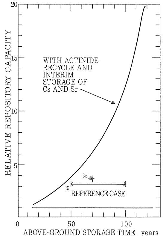
그림 3. 스트론튬 및 세슘의 군분리후의 지상보관 시간변화에 따른 지중매물 처분용량변화
