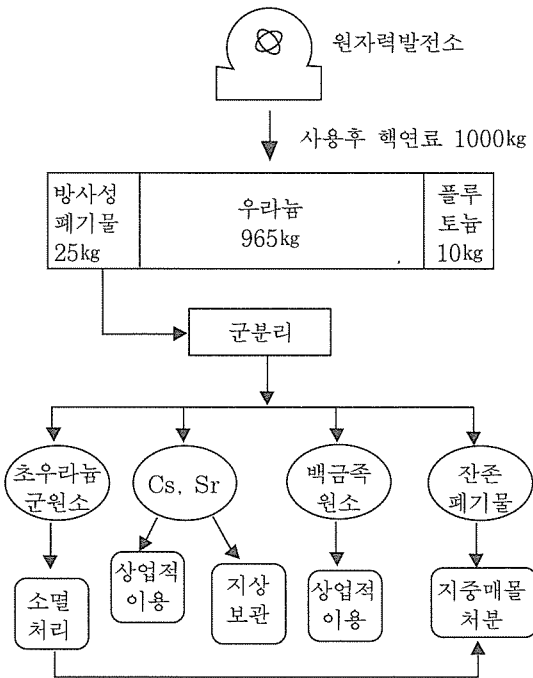
그림 1. 상용 고준위 방사성 폐기물의 군분리 개요
