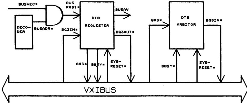
그림 4. 버스리퀘스터(Requestor)와 아비터(Arbitor)의 블록도 Fig. 4. Block Diagram of Bus Requestor & Arbitor
