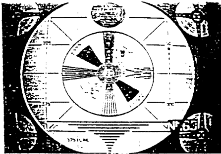
그림 14. 비완주사 Fig 14. The interlace scanning
