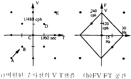
그림 3. 비월 주사방식에서의 샘플링 Fig 3. The Sampling of Interlace Scanning
