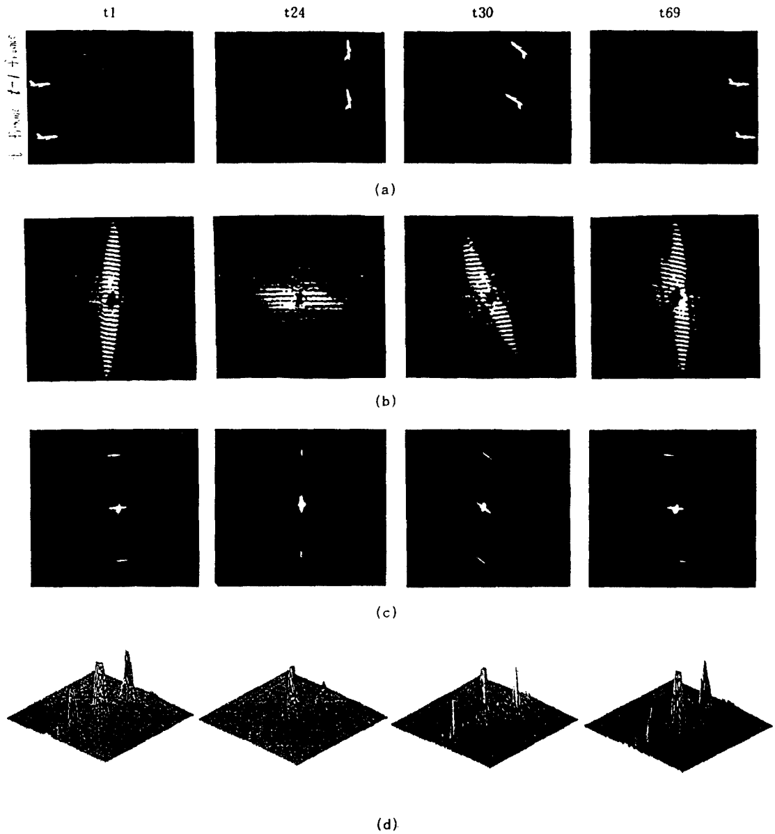
그림 6. Maneuvering하는 이동 표적에 대한 각 프레임 주기의 광 JTC 실험 결과
