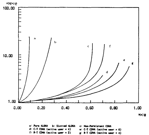
그림 14. 페이딩 잡음이 섞였을 때 채널 액세스 프로토콜의 트래픽양에 대한 지연시간(SNR=0 dB)
