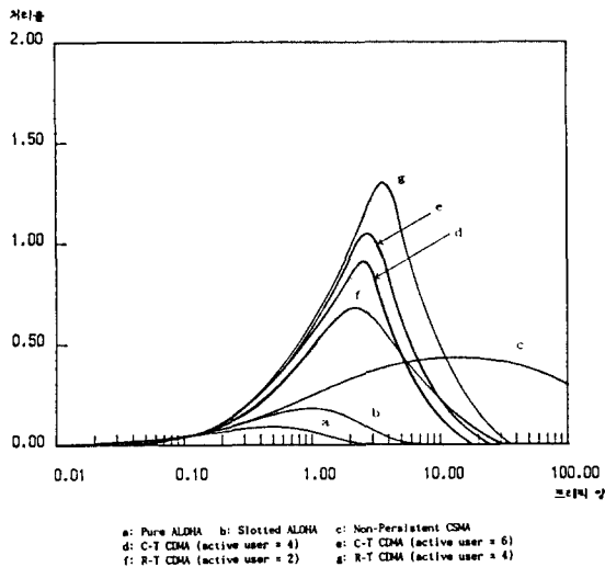
그림 12. 페이딩 잡음이 섞였을때 채널 액세스 프로토콜의 트래픽양에 대한 처리율 특성(SNR=0 dB)
