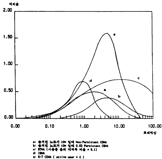
그림 10. 숨겨진 노드가 존재할 때 트래픽양에 대한 채널 액세스 프로토콜의 처리율 특성
