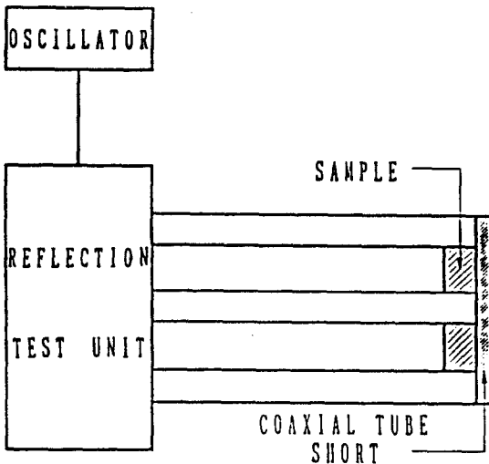
그림 3. 전파흡수능 측정장치 Fig. 3. Measurement Apparatus of Microwave Absorbing Characteristics.
