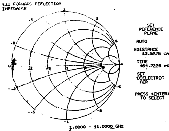
그림 5. Reference Plane을 단락판까지 이동시킨 때의 ADPT에 연결된 샘플홀더의 스미스도표상의 입력임피던스 Fig.5. Input Impedance on Smith Chart to the Sample Holder Connected with the ADPT When the Reference Plane is Shifted to the Shorted Plane.
