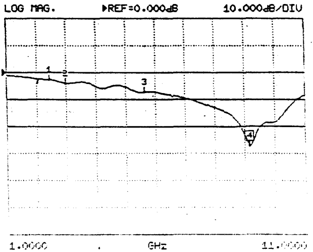
그림 7. 제작된 샘플홀더 및 ADPT.3에 의하여 측정된 전파흡수체(샘플; C-1)의 전파흡수 주파수특성
