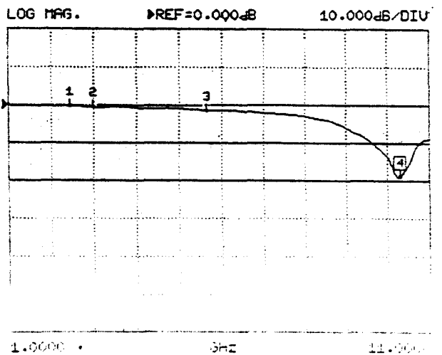
그림 8. 제작된 샘플홀더 및 ADPT.3에 의하여 측정된 전파흡수체(샘플; C-2)의 전파흡수 주파수특성
