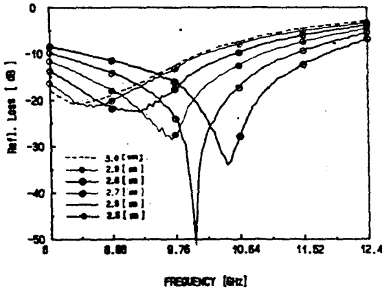
그림 13. 측정된 재료정수(그림12(a) 및 (b))로부터 계산된 샘플C-1의 전파흡수 주파수특성
