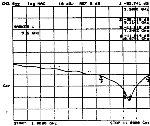
그림 9. 7mm \phi Air Line에 의하여 측정된 전파흡수체(샘플; C-1)의 전파흡수 주파수 특성
