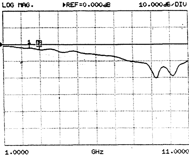
그림 6. ADPT와 샘플홀더에 의하여 측정된 전파흡수체 시편(샘플; A-1)의 전파흡수 주파수특성
