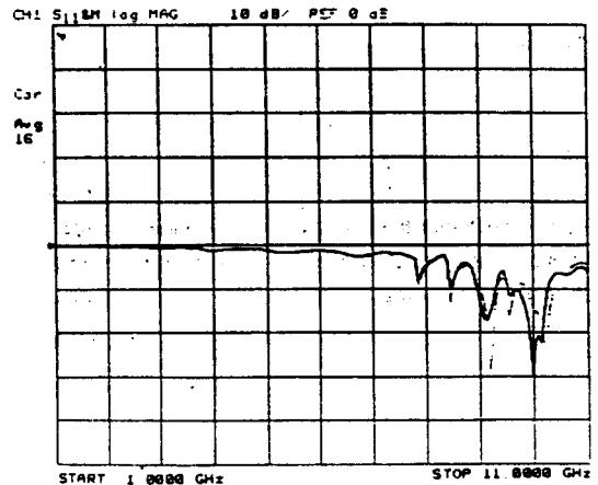
그림 11. X-Band용 구형도파관에 의하여 측정된 샘플 C-2의 전파흡수 주파수 특성
