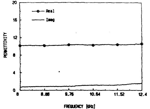
그림 12(b). 측정된 샘플C-1의 복소 유전율 Fig. 12(b). Measured Relative Permittivity of Sample C-1.
