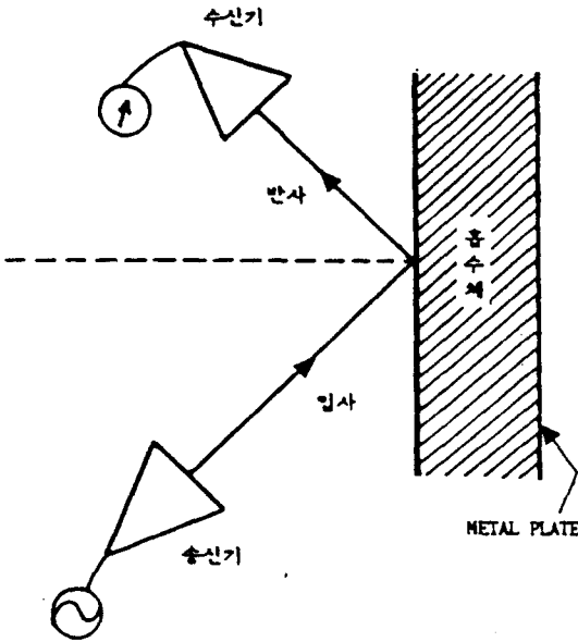
그림 2. 반사전력법 Fig. 2. Reflected Power Method.
