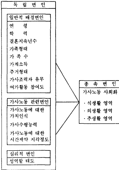
(그림 1) 연구모형
