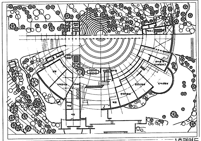
1층평면도
