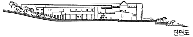
단면도
