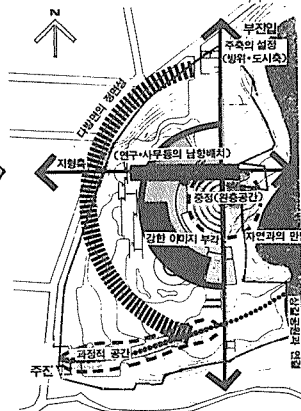
배치개념도
