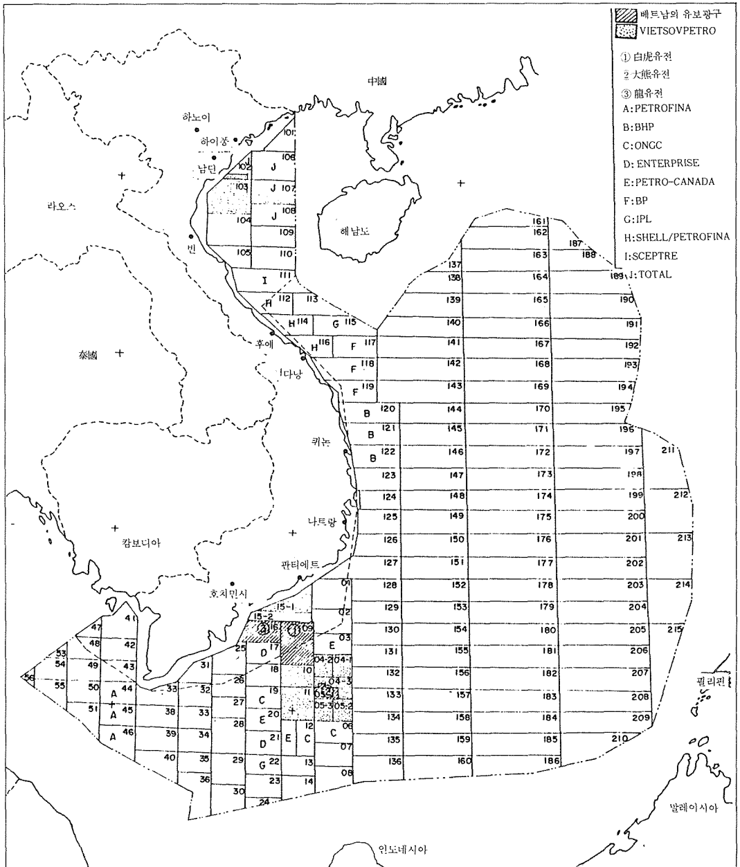
〈그림-1〉 베트남의 대륙붕 광구 현황
