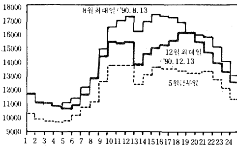
'90년 동·여름 최대부하일 부하곡선
