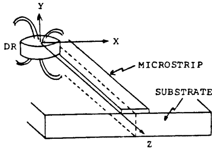
그림 3. 마이크로스트립 선로상의 공진기 Field Magnetic flux linkage Magnetic flux linkage of the resonator into the microstrip line
