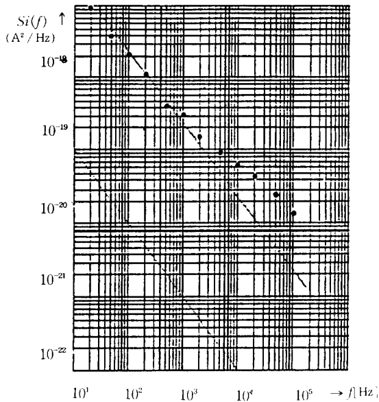
그림 6j. GaAs(100), n'-type, R=497Ω, I x =9.37mA
