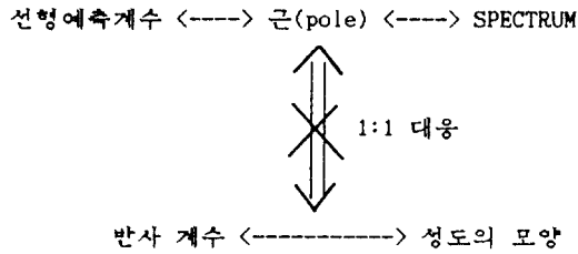
그림 7. 선형예측계수와 성도의 모양과의 관계 Fig. 7. Relation between LPC and vocal tract shape
