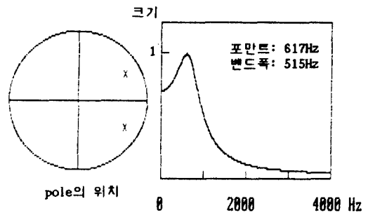
(a) 2 pole일 때
