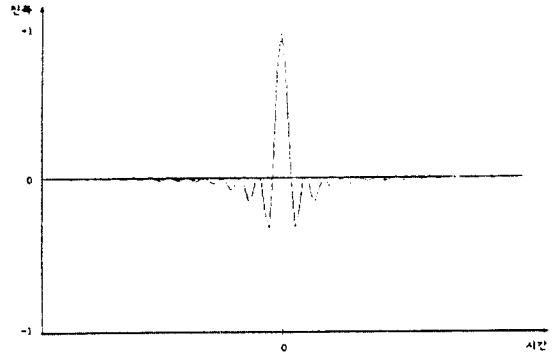
그림 5. 전화신로의 모델 I에 대한 임펄스 응답 Fig. 5. The impulse response of the model I for the telephone channel.
