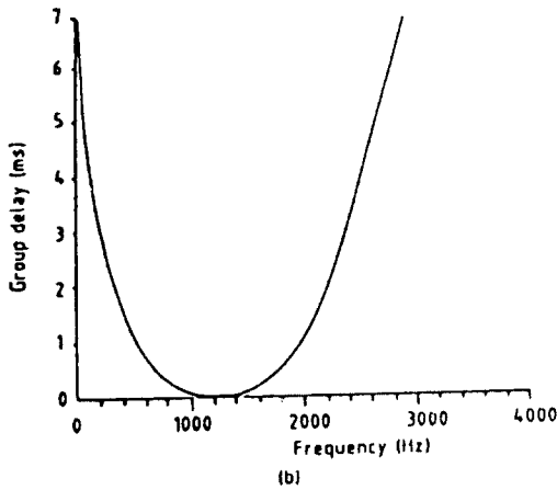
그림 4. 전화신로의 모델 V에 대한 주파수 특성 (a) 진폭 특성 (b) 지연 특성 Fig. 4. The frequency response of the model V for the telephone channel. (a) The amplitude characteristics (b) The delay characteristics
