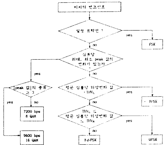
그림 7. 위상차의 peak값을 이용한 모델 형태의 식별 흐름도. Fig. 7. The flowchart for the classification algorithm of the modulation type using the phase difference and peak value.
