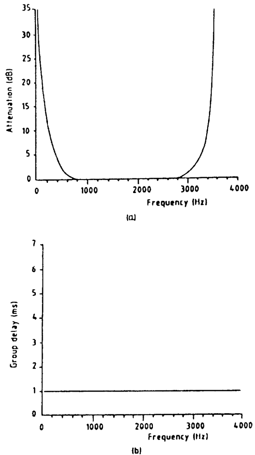
그림 3. 전화선로의 모델 1에 대한 주파수 특성 (a) 진폭 특성 (b) 지연 특성
