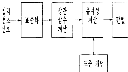
그림 8. 상관함수를 이용한 모델 형태의 판별 블록도 Fig. 8. The block diagram for the classification algorithm of the modulation type using the correlation characteristics.
