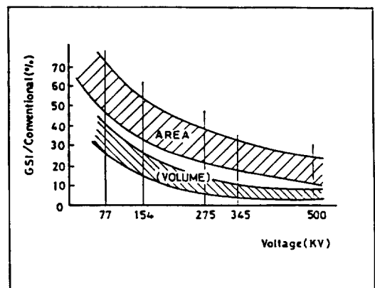
그림 1. 변전소 설치면적 및 비교표
