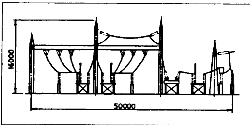
그림 3. 옥외철구형 변전소 단면도
