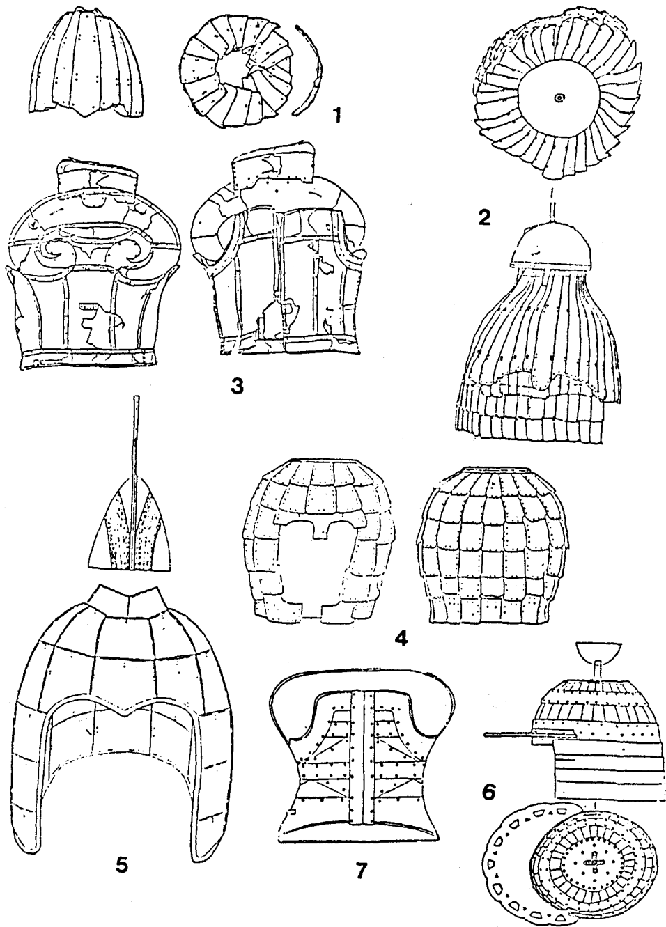
<第4圖> 영남지방 4, 5세기대의 갑주(1: 예안리 150호분 투구, 2: 복천동 11호분 투구, 3: 복천동 10호분 단갑, 4: 중국 화국성 연화도 제44호분 소찰혁철 투구, 5: 함천 반계제 가-A호주분 투구 복원도, 6: 동래 연산동, 7: 함양 상백리 고분)
