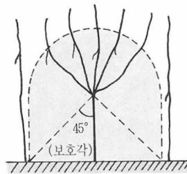
피뢰침의 효과
