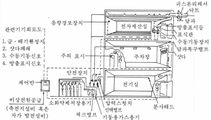
<그림 1> 가스 소화 설비 계통도
