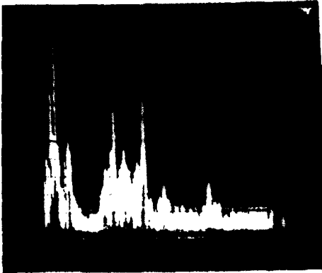
Photo. 3 Rcp 2 mm Notch (H : 10 \mu s / div, V : 50mv / div)
