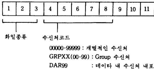
Fig. 6 시스템에서 사용하는 파일명의 구성
