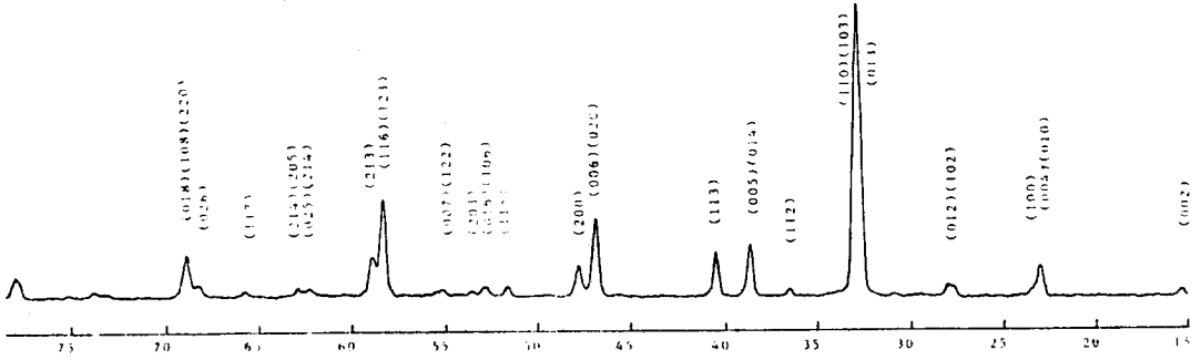
그림 5. 하소분말의 x-ray회절분석
