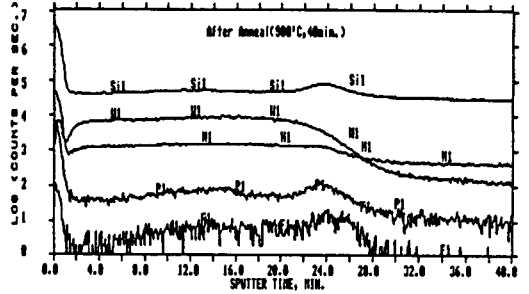
그림 11. 900°C, 40min. annealing 후 WSi_x ( WF_6=16SCCM )막의 SIMS depth profile.
