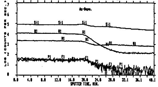
그림 10. As-deposited WSi_x ( WF_6=16SCCM )막의 SIMS depth profile.
