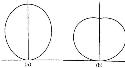
그림 11. (a) Tb의 overcosine 방출분포
