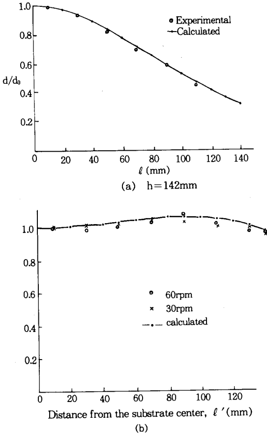
그림 4. 코사인분포법칙과 환상타겟 가정에 의한 두께분포의 계산치와 실험치의 비교:(a) 기판정지, 전극간거리 142mm (b)기판회전
