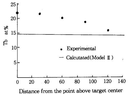
그림 7. 조성분포의 실험치 및 모델 II의 계산치 Fig 7. Experimental and calculated composition profiles using Model II.
