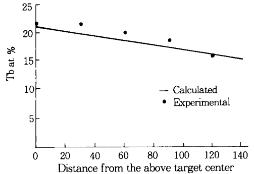
그림 10. Tb(overcosine), Fe(undercosine)의 방출분포를 고려한 계산치와 실험치의 조성분포 비교
