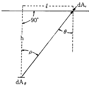
그림 2. 미소평면 source에서 평행평면 기판에의 증착
