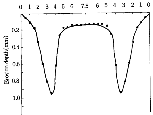
그림 5. 원판형 마그네트론 타겟의 반경방향의 침식분포
