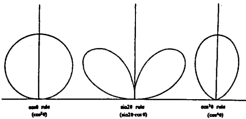
그림 8. \cos\theta, \sin 2\theta 및 \cos^3\theta 방출분포 Fig 8. Emission profiles for cosine( \cos^2\theta ), undercosine ( \sin 2\theta ) and overcosine( \cos^3\theta ) emission.
