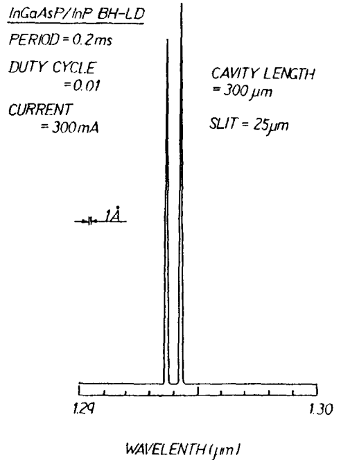
그림 10. InGaAsP/InP BH-LD의 스펙트럼.
