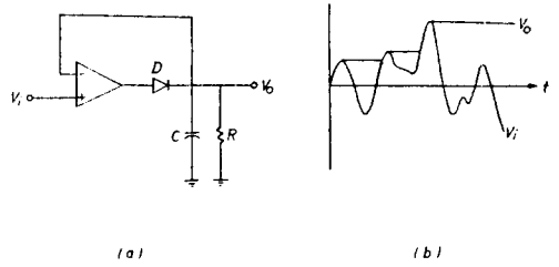
그림 5. 최대값 검출기의 원리. (a) 최대값 검출기의 기본회로, (b) 최대값 검출기의 입·출력 관계
