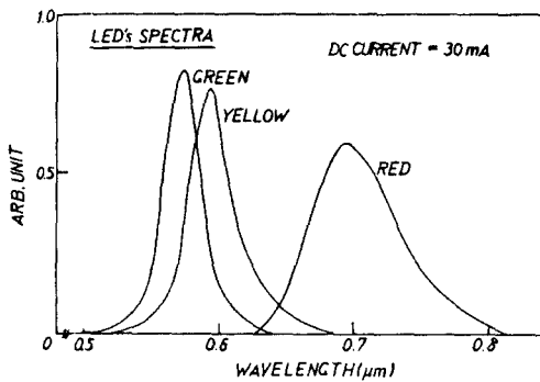
그림 7. 직류구동상태의 LED의 스펙트럼.
