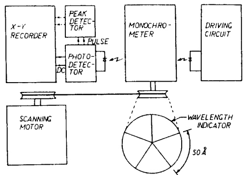
그림 2. 분광기를 이용한 파장분석 장치.
