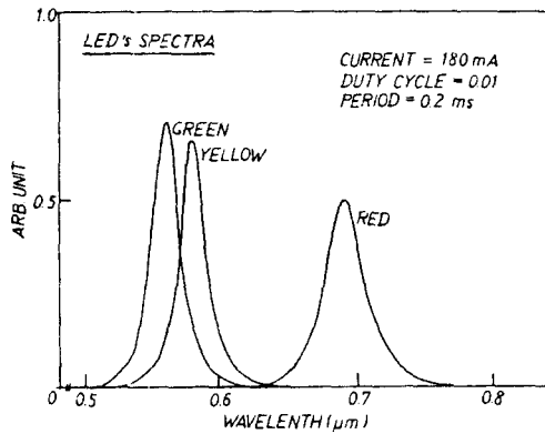
그림 8. 펄스구동상태의 LED의 스펙트럼.
