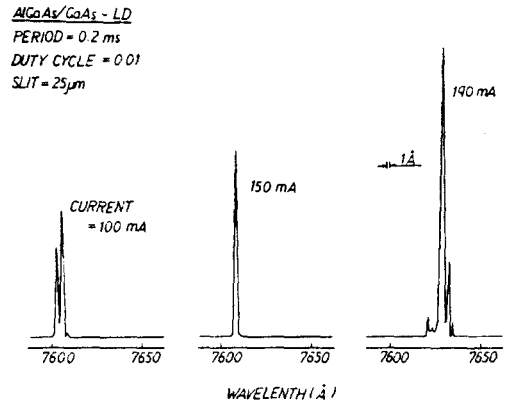
그림 9. AlGaAs/GaAs LD의 스펙트럼.
