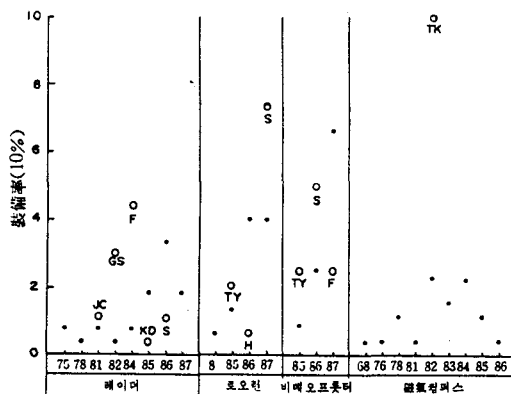
그림 6. 集魚船의 航海用 電子機器의 製作年度 및 製作會社別 裝備率.
