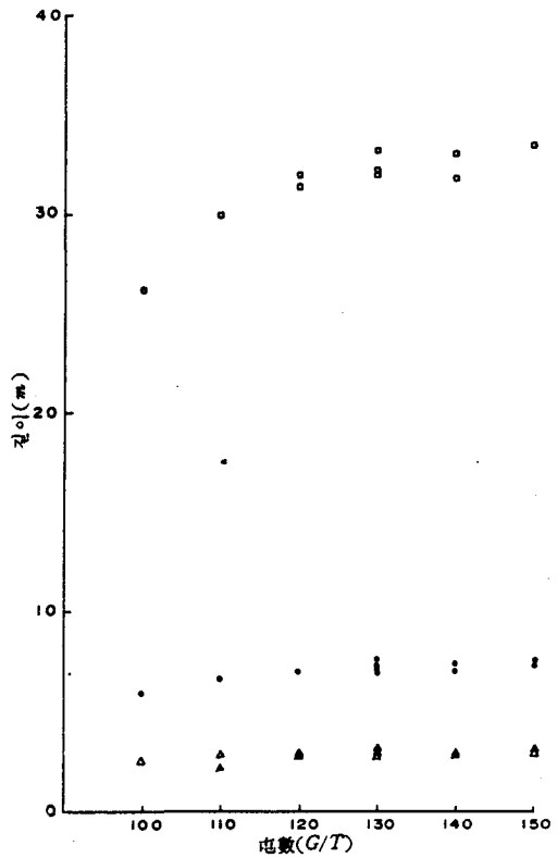
그림 2. 本船의 屯數級別 全長, 全幅, 船의 깊이.
