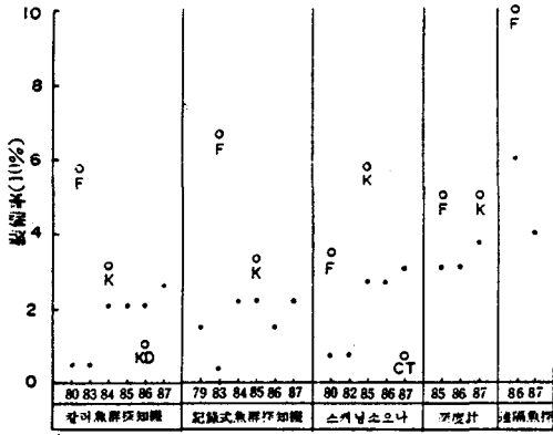
그림 3. 本船의 漁撈用 電子機器의 製作年度 및 製作會社別 裝備率. F : 古野電氣, K : 海上電氣 KD : Koden, CT : C. Tech.
