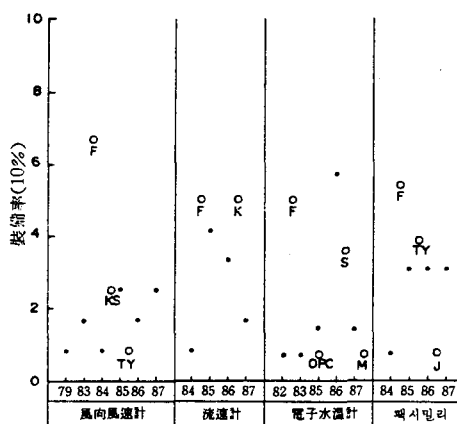
그림 7. 本船의 氣象·海象觀測用 電子機器의 製作年度 및 製作會社別 裝備率.
