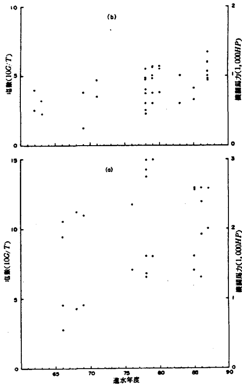
그림 1. 本船 및 集魚船의 進水年度別 屯數 및 機關馬力.
