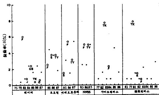
그림 5. 本船의 航海用 電子機器의 製作年度 및 製作會社別 裝備率
