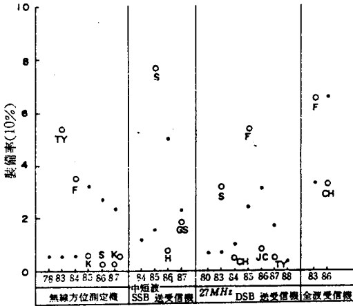
그림 9. 集魚船의 通信用, 電子機器의 製作年度 및 製作會社別 裝備率.
