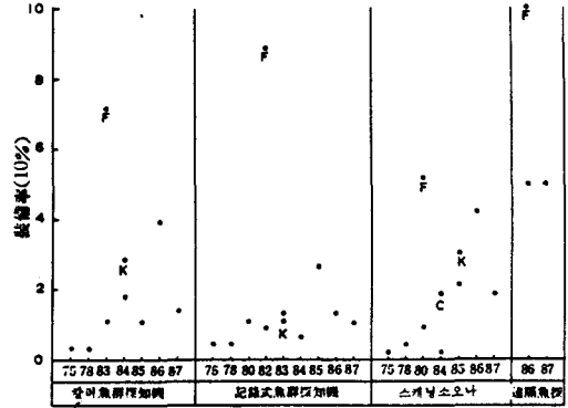
그림 4. 集魚船의 漁撈用 電子機器의 製作年度 및 製作會社別 裝備率 F : 古野電氣, K : 海上電氣, C : C. Tech.
