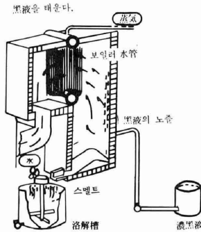
〈보일러의 構造〉
