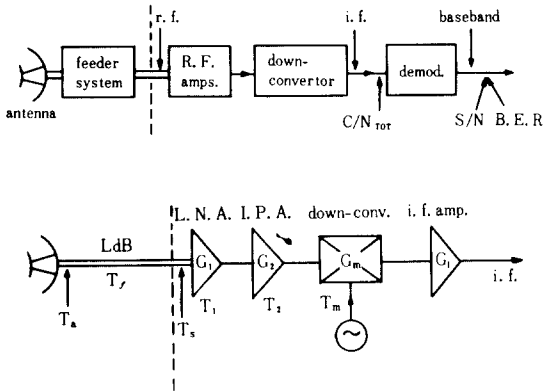
그림 1. 수신기 계통도 및 잡음온도 계산
