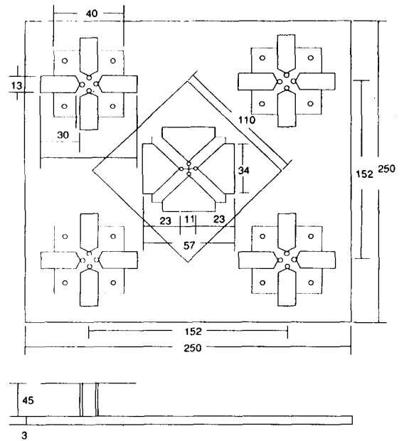
그림 4. 신호수신(중앙) 및 4개의 monopulse 추적용 안테나
