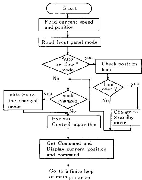
그림 9. 운용 프로그램의 흐름도
