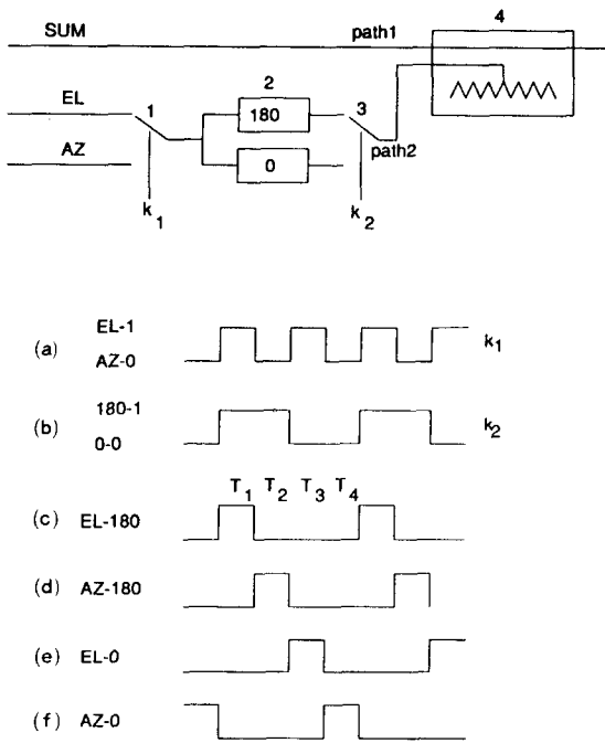
그림 3. 단일 주사 변환기의 신호처리 시간흐름도
