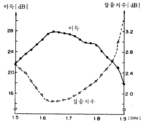
그림 7. 저잡음 증폭기 특성
