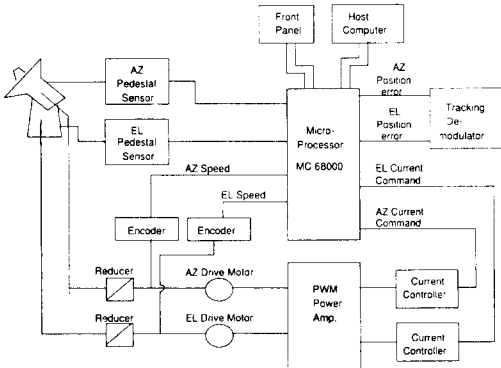
그림 8. 안테나 구동 시스템 계통도
