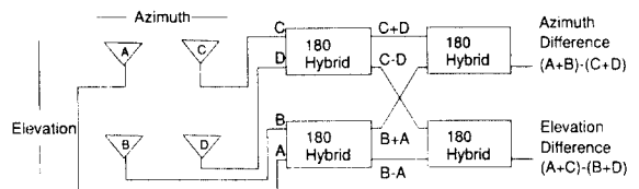
그림 2. Monopulse 시스템으로 4개의 안테나 및 4개의 hybrid
