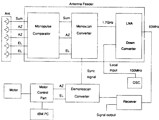
그림 5. 수신 시스템 계통도
