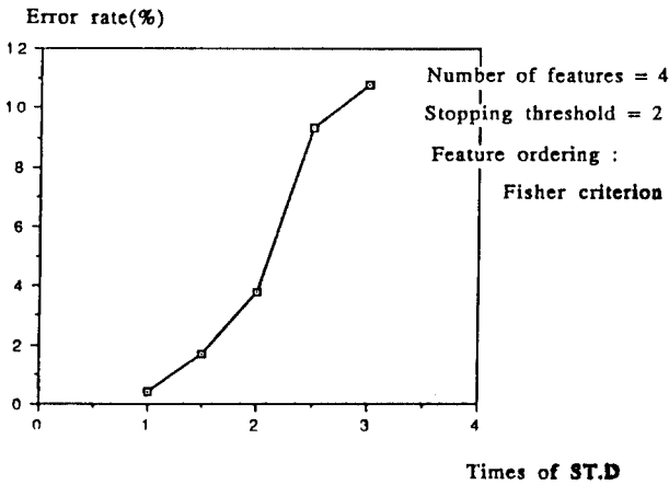
그림 10. 특징의 표준 편차와 오인식률의 관계 The relation between standard deviation and error rate
