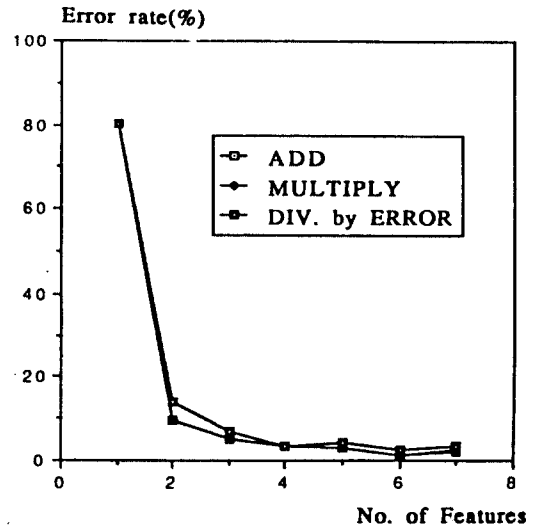
그림 7. 제안한 여러가지 criterion에 대한 오인식률 Error rate of the proposed classification algorithm
