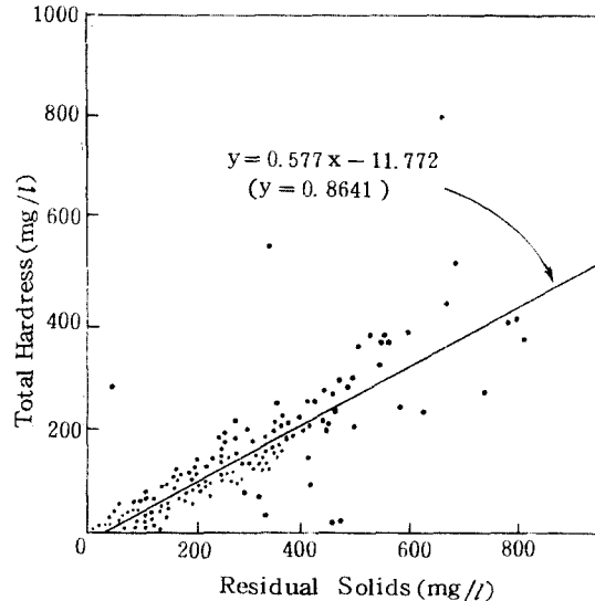
Fig. 1. The Estimated Regression Line of R. S. and T. H.
