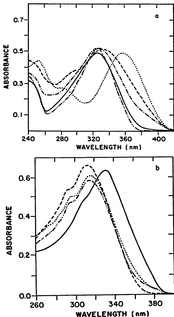
Figure 1. Absorption spectra of piroxicam and HMBDC in various solvents: (a) 4.0 \times 10^{-5} M solution of piroxicam: (---) n-hexane; (---) dioxane; (---) butanol; (---) ethanol; (.....) H_2O . (b) 5.0 \times 10^{-5} M solution of HMBDC. (---) n-hexane; (---) butanol; (.....) methanol; (---) H_2O .
