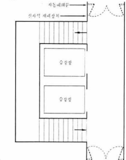
그림 3 : 기존통로에 설치된 방연문
