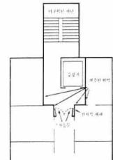
그림 6 (b) : 개수후의 계단과 승강로
