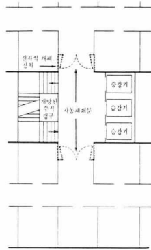
그림 4 : 승강기와 계단실을 구획하기 위한 방연문의 설치
