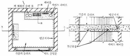
닥트 단면도
