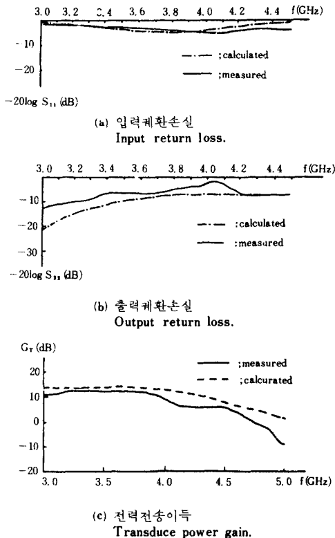
그림12 주파수에 대한 입출력 제환손실과 이득 I/O return loss and gain vs. frequency response.
