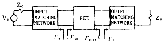
그림 1 증폭기 계통도 Amplifier block diagram.
