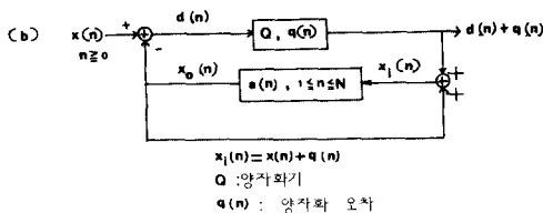
(b) N차 선형 예측기를 사용한 DPCM의 블럭도 (b) Block diagram of DPCM using Nth order linear predictor
