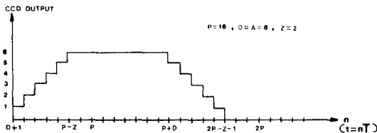
그림 7 식(11)분산형 마스크를 사용할 경우의 임펄스 응답. Impulse response with the dispersive mask (11).
