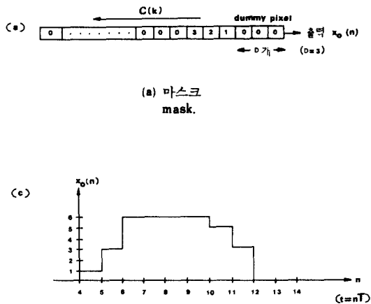
(b) CCD 내부신호 분포 CCD pixel signal distributions.
