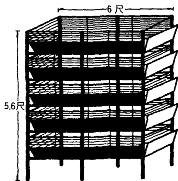
● 幼雛用 케이지 5段 10室
