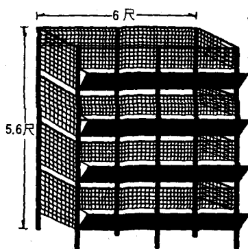
● 中雛用 케이지 4段 8室
