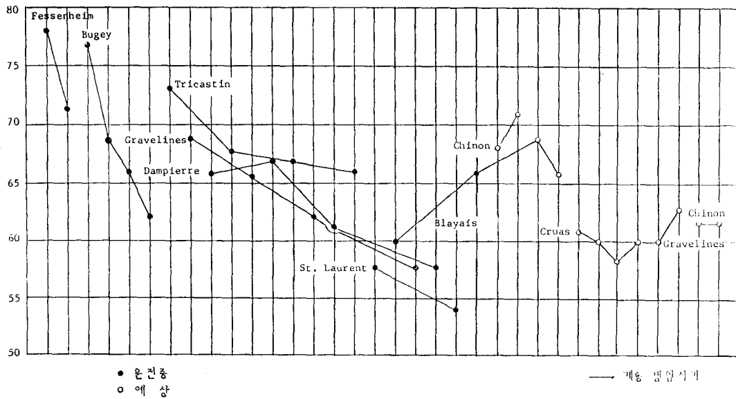
그림 3. 프랑스 900MWe급 표준발전소 建設기간(원자로 발주에서 계통 병입까지)
