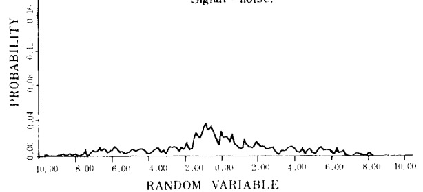
그림 10 신호+잡음의 확률밀도함수 pdf of signal + noise.
