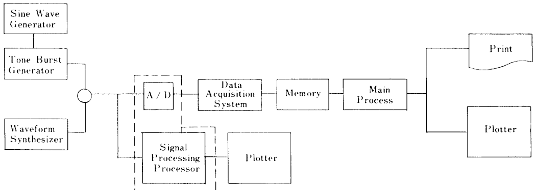
그림 4 信号처리를 위한 全体 시스템 구성 Whole system block for signal processing.
