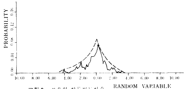
그림 8 잡음의 확률밀도함수 pdf of noise.
