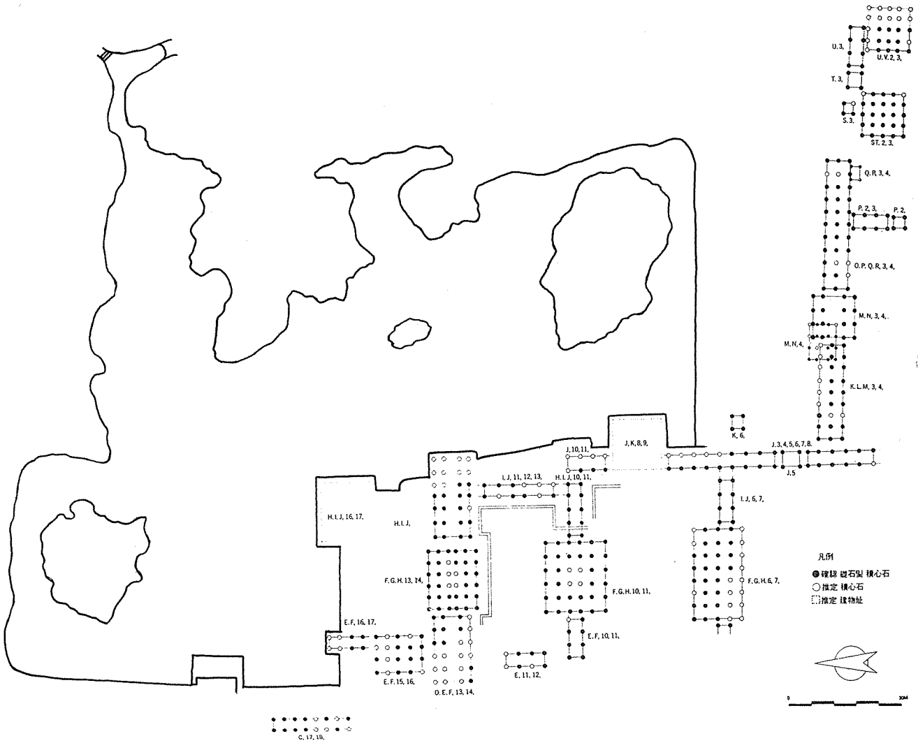
圖 2 : 경주 안압지 주변 建物址 (통일신라시대)
