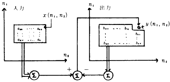
그림 1 식(2)에 의한 필터의 수행과정 Diagram of how the output is completed.
