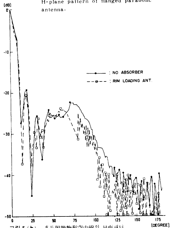
그림 5 (b) 후드附拋物形空中線의 H面패턴 H-plane pattern of Hooded parabolic antenna.
