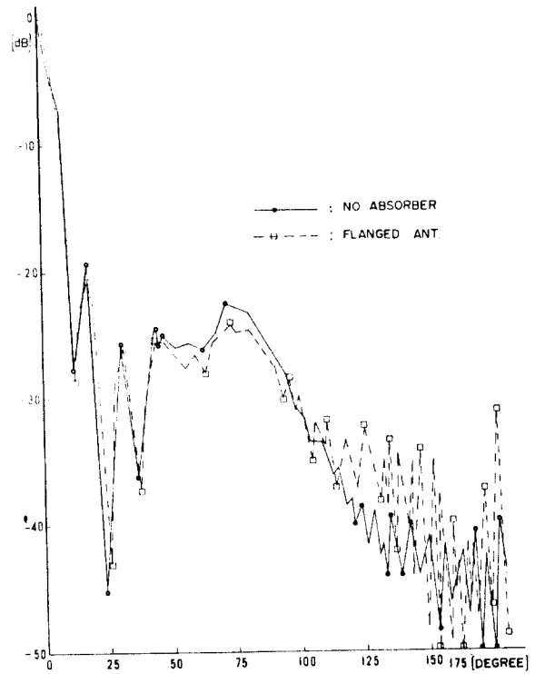
그림 4 (b) 水兵帽形테드리附 拋物形空中線의 H面패턴 H-plane pattern of flanged parabolic antenna.
