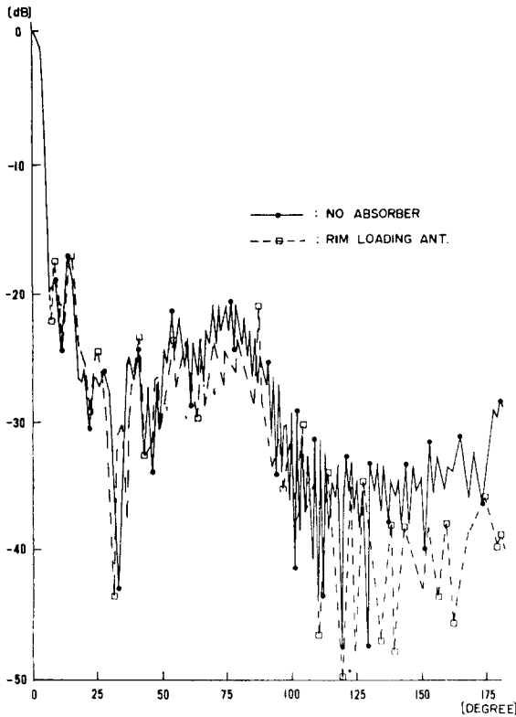
그림 3 (a) 周邊裝荷拋物形空中線의 E面패턴 E-plane pattern of side rim loading parabolic antenna.
