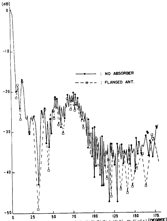
그림 4 (a) 水兵帽形테드리附 拋物形空中線의 E面패턴 E-plane pattern of flanged parabolic antenna.
